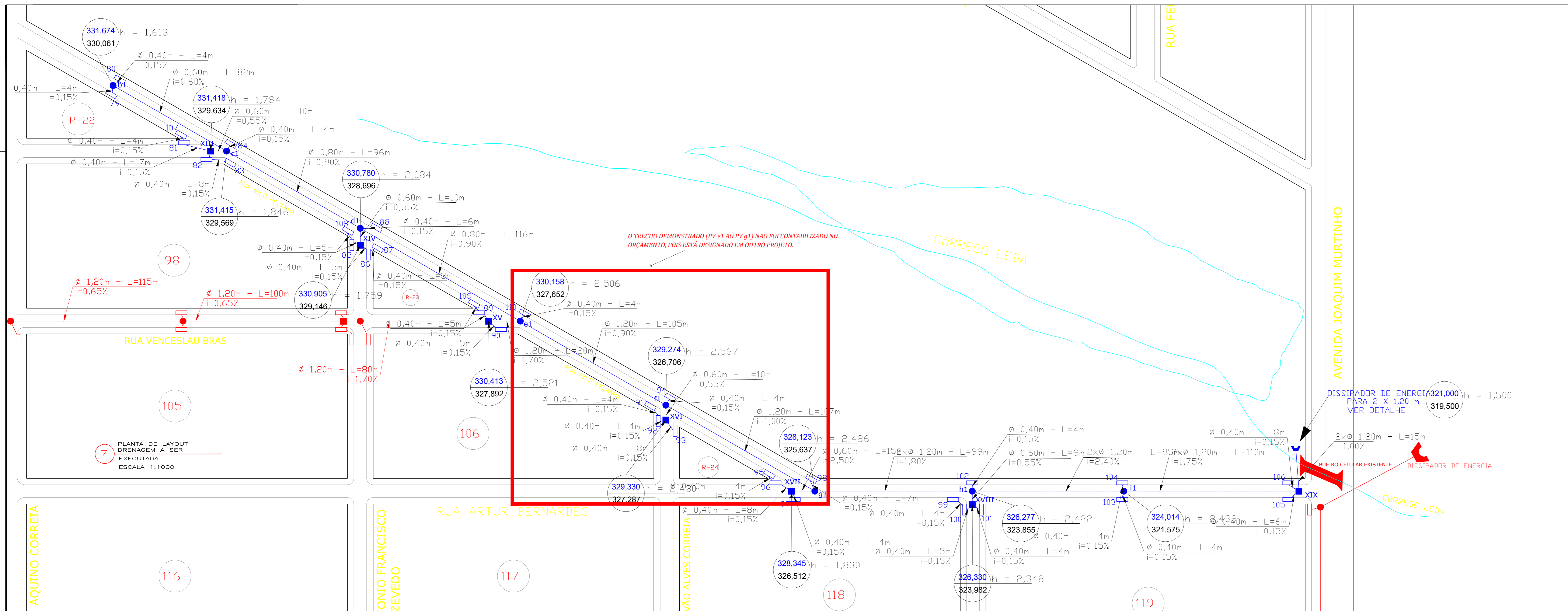
7 PLANTA DE LAYOUT DRENAGEM A SER EXECUTADA ESCALA 1:1.000
