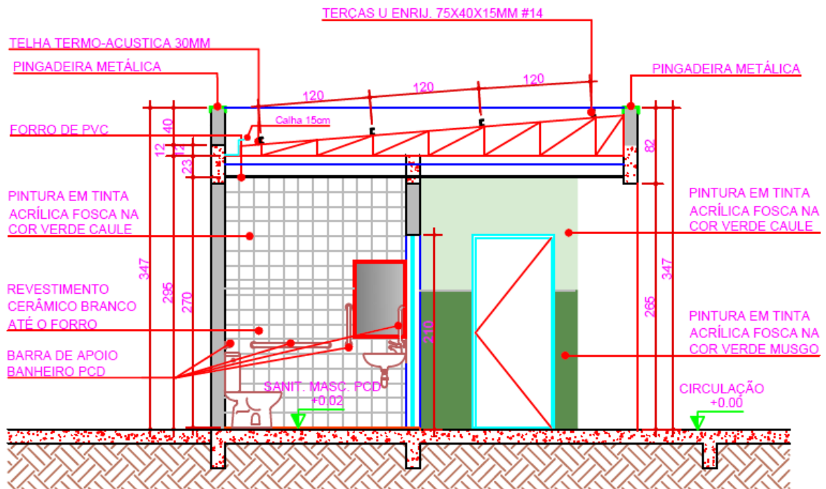
Figura 5 Corte AA Banheiros
