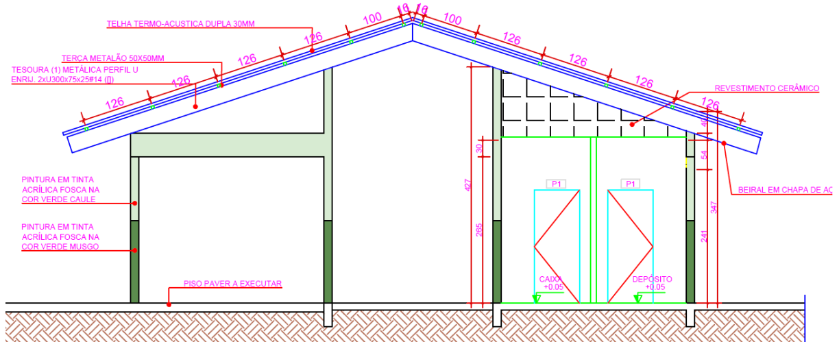
Figura 3 Corte AA
