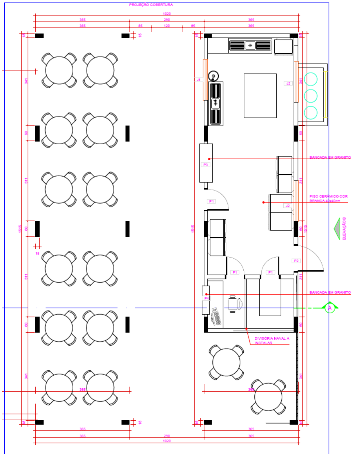
Figura 2 Planta baixa Cozinha
