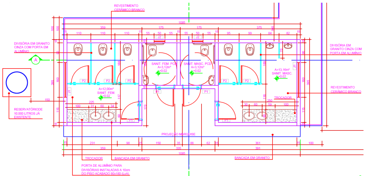
Figura 4 Planta Baixa Banheiros
